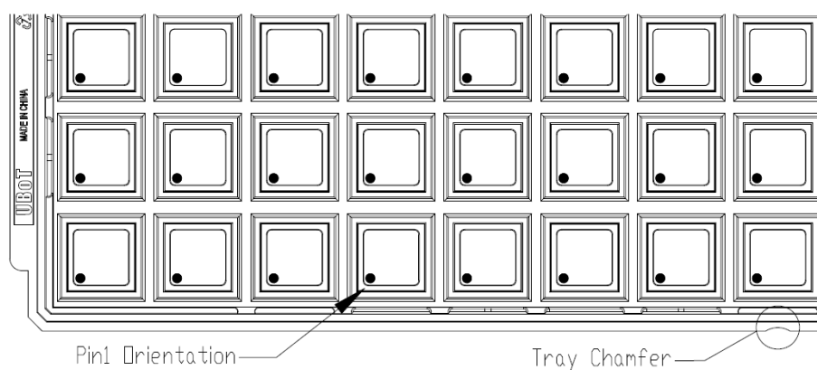
图 25 托盘包装示意图
