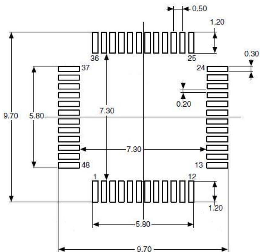
图 22 LQFP48, 7×7mm 焊接 Layout 建议
