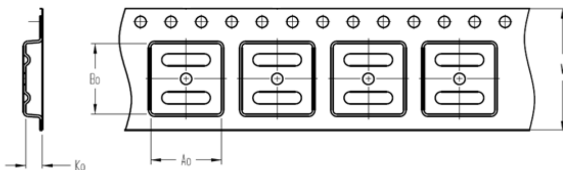
图 24 带状包装规格图
