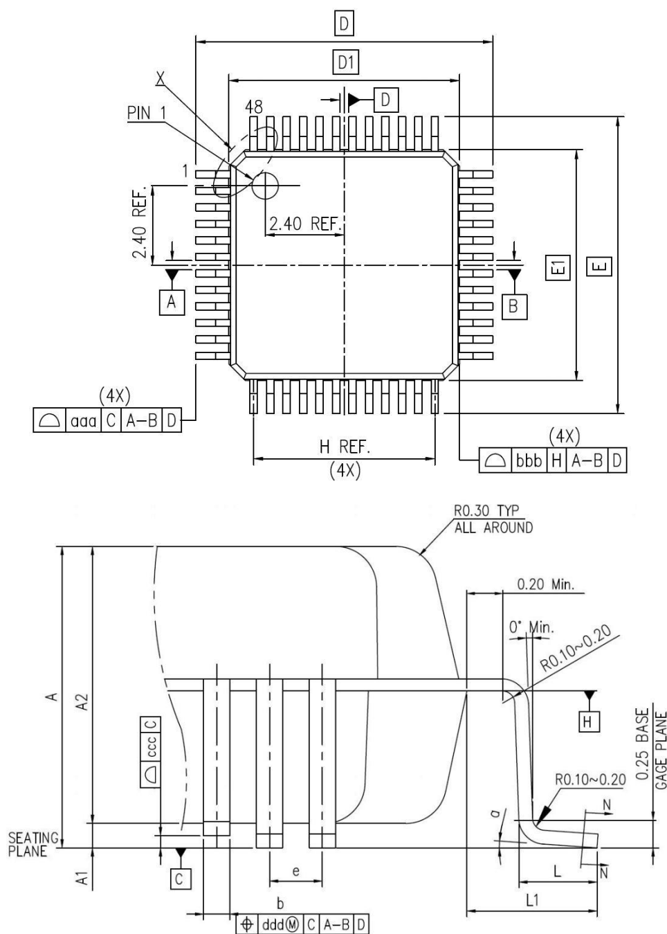
图 21 LQFP48 封装图
