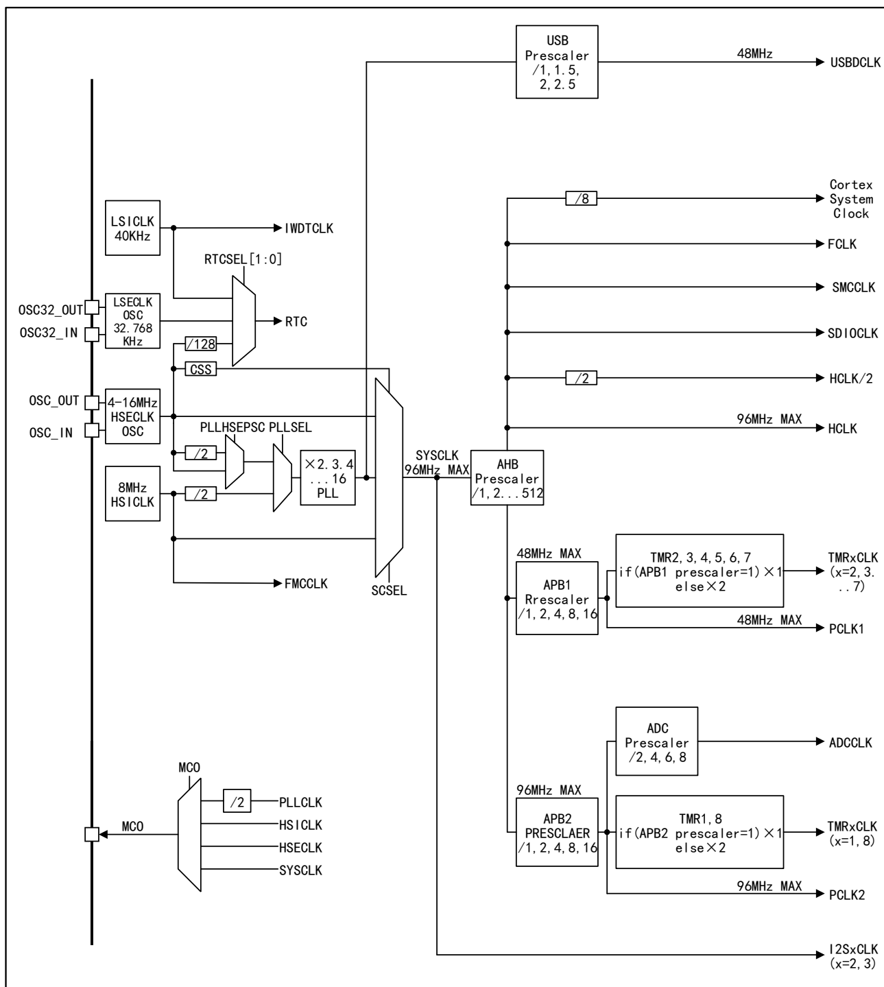
图 7 APM32F103xC 时钟树
